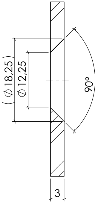
SCHNITT B-B MAßSTAB 2 : 1
